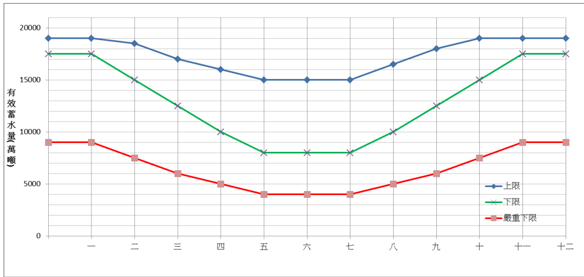
附圖 石門水庫運用規線圖
